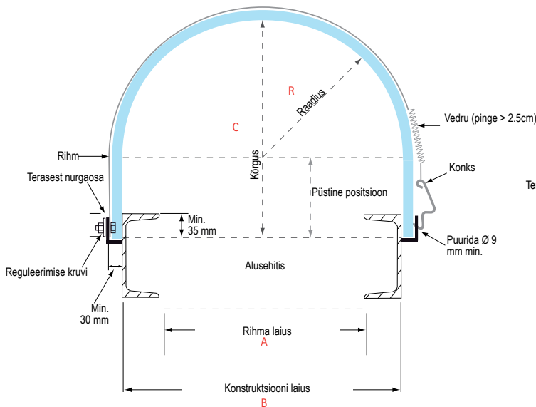
Rihmaga kinnitamine katetele n° 1-2-3-4
