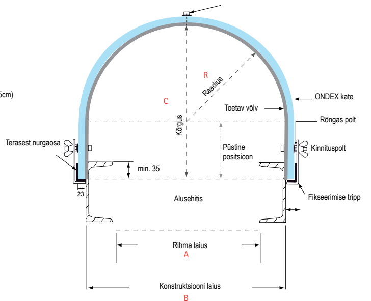
Võlviga kinnitamine katetele n° 5 ja edasi
