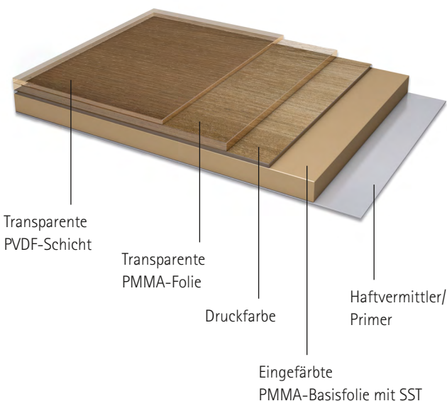
Schematischer Aufbau der Außenfolie RENOLIT EXOFOL FX
