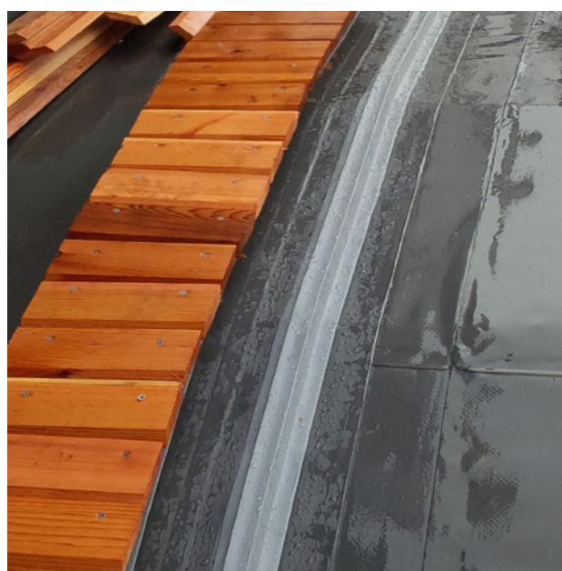
Les pièces d'habillage en bois sont fixées sur des profilés RENOLIT ALKORPLAN Solar
